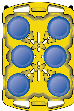
ADD6 Diseño para platos de 21,28 cm a 24,76 cm
